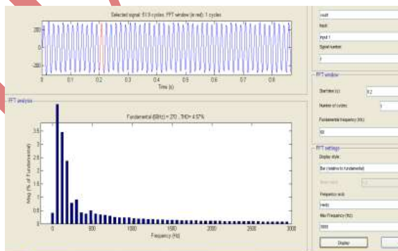
Fig: 13 THD
