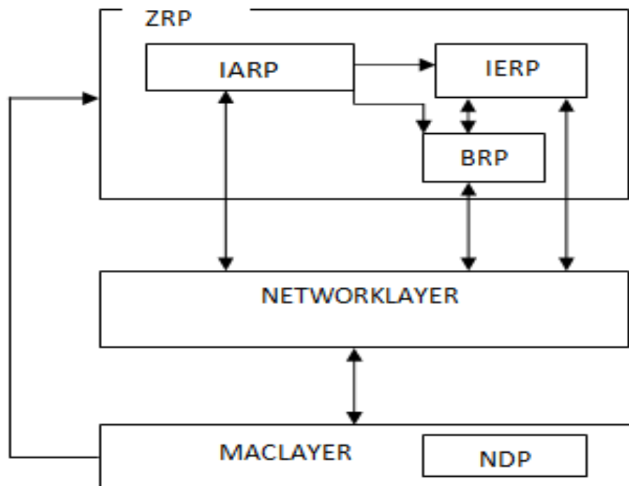
Fig:ZRPArchitecture
